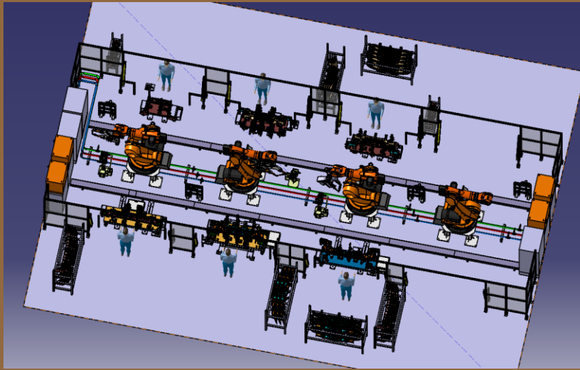
重庆明天机械长安 B561、C281尾裙板 焊接集成项目
