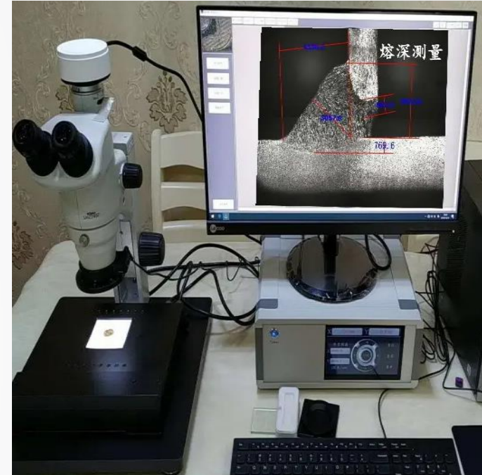
焊接溶深检测
