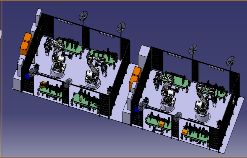
重庆卓通长城P01 焊接工作站集成项 目
