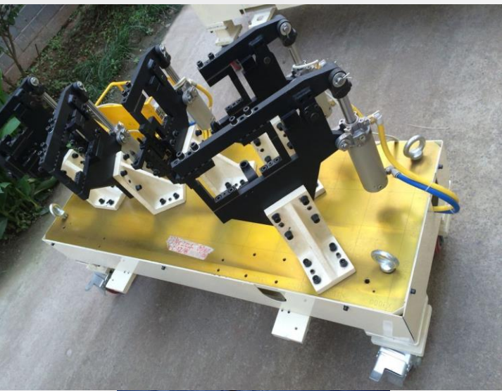
焊接工装展示
