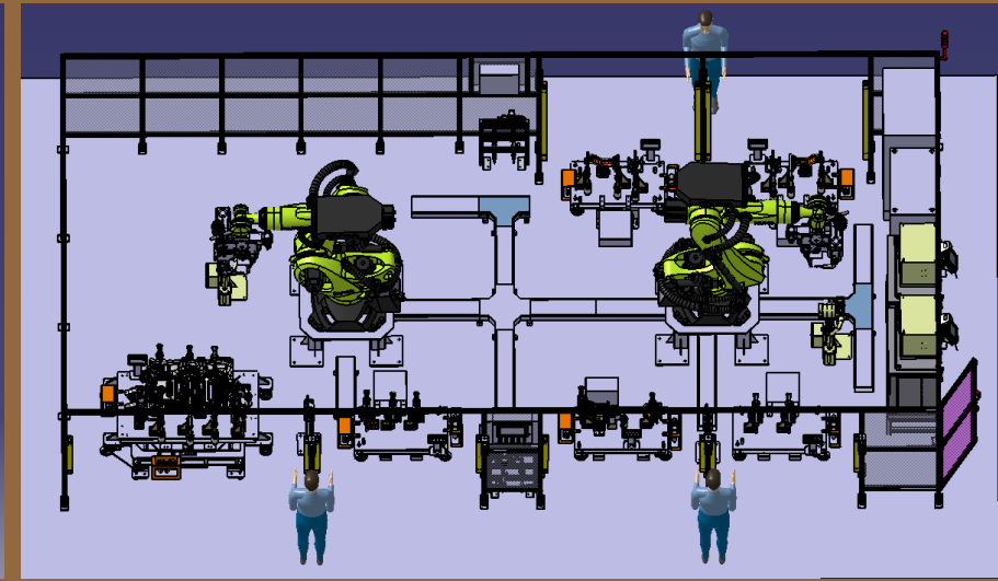
重庆澳腾长城P027 焊接工作站集成项 目
